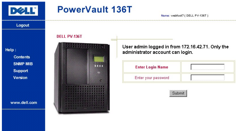
Abbildung 7. Dialogfeld "Login"
